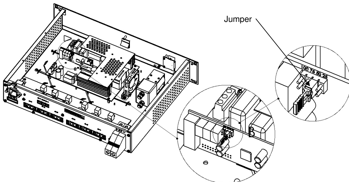
Bild 1 : Jumperlagebestimmung
