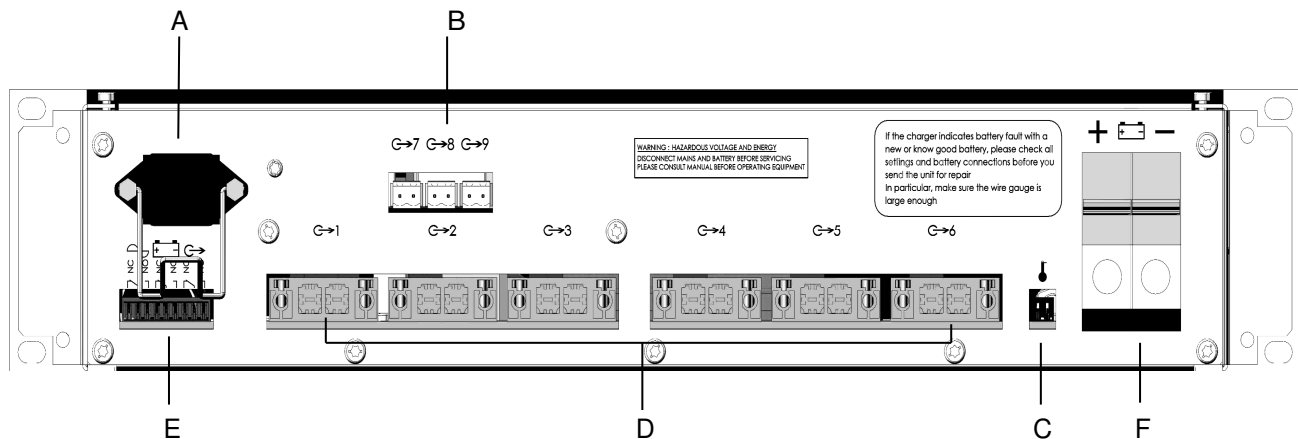
Bild 5 : Rückseite
