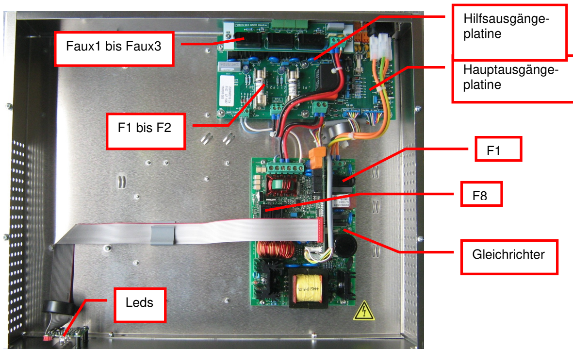
Bild 1 : Innenansicht
