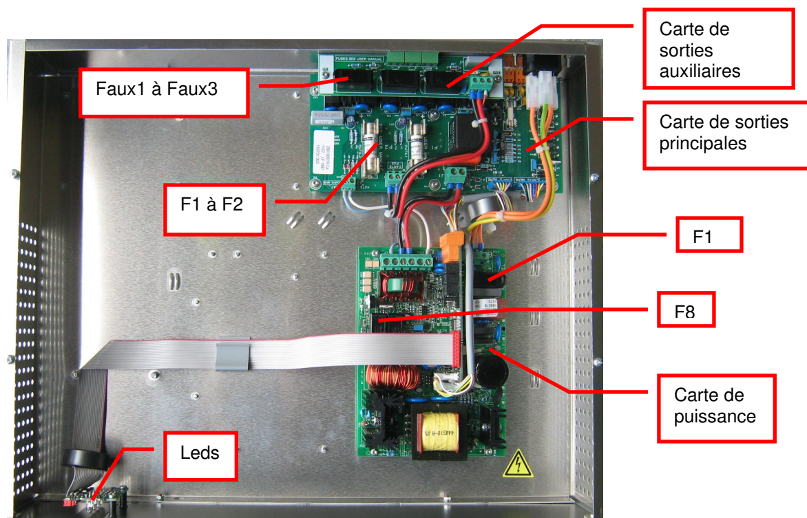
Figure 1 : vue interne
